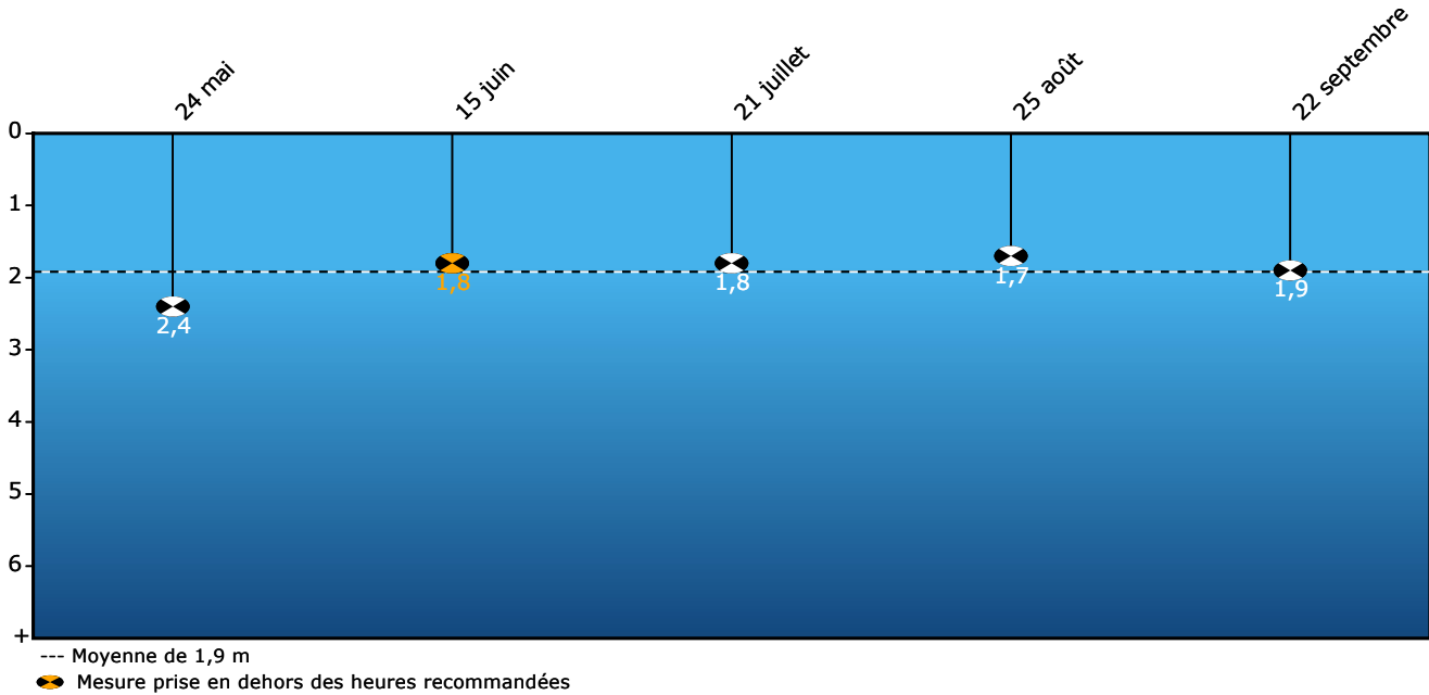
Transparence de l'eau - Été 2009 (profondeur du disque de Secchi en mètres)
